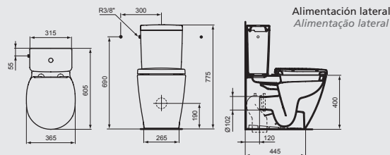
Inodoro con depósito Arco / Bacia com tanque Arco
