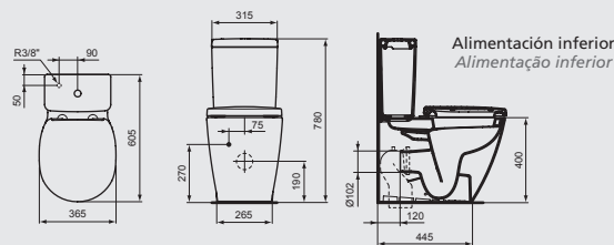
Inodoro con depósito Cúbico / Bacia com tanque Cúbico
