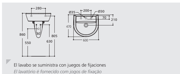
El lavabo se suministra con juegos de fijaciones El lavatório é fornecido com jogos de fixação
