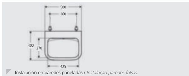
Instalación en paredes paneladas / Instalação paredes falsas
