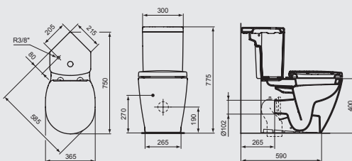
Inodoro con depósito Angular / Bacia com tanque Angular
