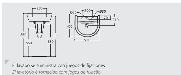
El lavabo se suministra con 2 juegos de fijaciones El lavatório é fornecido com 2 jogos de fixação
